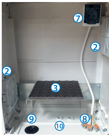
Figure 4 - Vue d'intérieure de l'armoire
